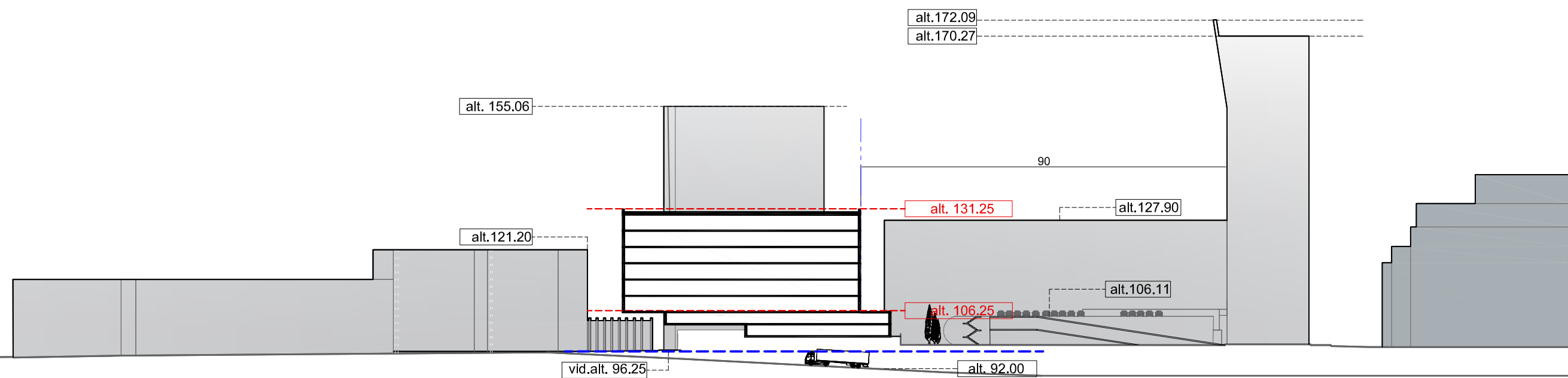
Išilginis pjūvis per Geležinio Vilko g.
